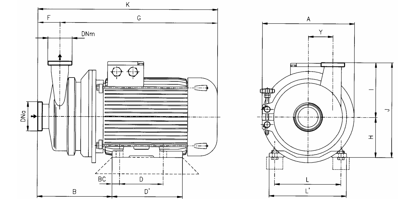
Размеры могут изменяться. DN = арматура с внутренней резьбой по DIN 11851
